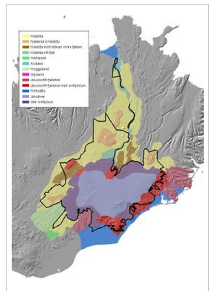
Mynd 3.6: Meginlandslagseiningar Vatnajökulspjóðgarðs
