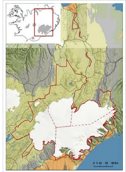
Mynd 3.5: Helstu jarðmyndanir á austurhluta Íslands. Grænleitt: Blágrýtismyndunin (16–3.3 milljónir ára) Blágrátt: Grágrýtismyndunin (3.3 – 0.8 milljónir ára) Gult: Móbergsmyndunin (0.8– 0.015 milljónir ára) Rauðgult: Laus jarðlög frá nútíma
